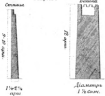
Разрѣзь
