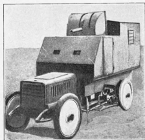
Фиг. 10. Скорострѣльная пушка 5 см. на бронированномъ автомобиль системы Эрхарда.
