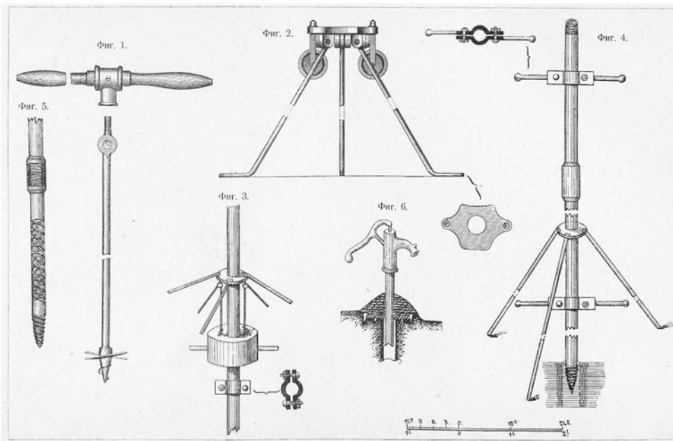
Фиг. 1—развѣдочный буръ; фиг. 2, 3 и 4—треноги для забивки и завинчивания трубы; фиг. 5—колодези. наконечникъ; фиг. 6—насосъ.
